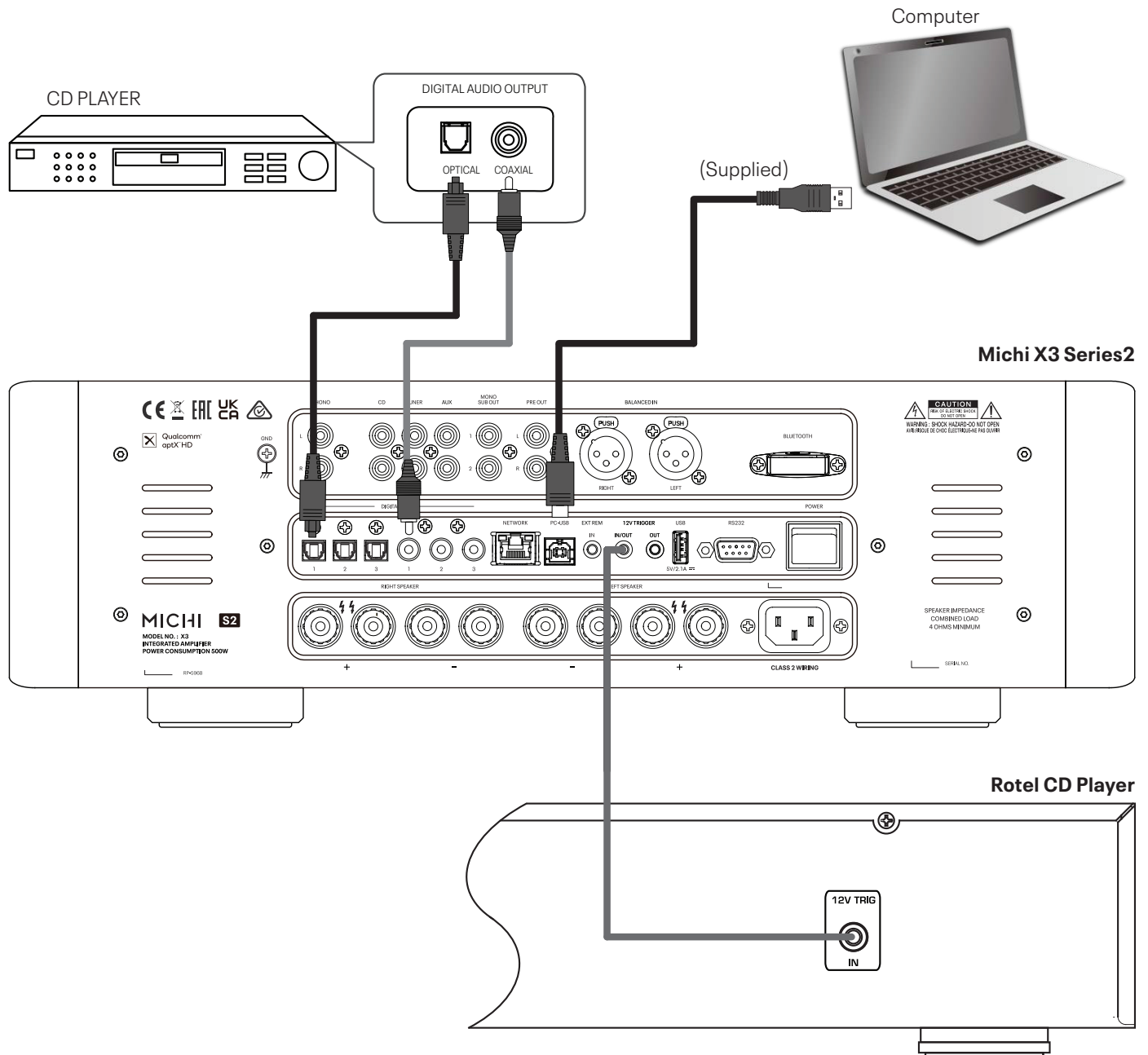
Figure 4: Digital Input and 12 Volt Trigger Connections Entrées numériques et Branchements des trigger 12 V Anschlussdiagramm (Digitaleingänge, 12V-Trigger) Entrada Digital y Conexiones para Señal de Disparo de 12 Voltios Digitale ingangen en 12V-trigger Collegamenti ingressi digitali e segnali Trigger 12 V Anslutningar för digitala ingångar och 12-volts styrsignaler Цифровой вход и выход 12-В триггерного
