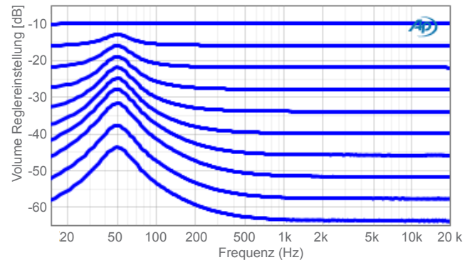
Frequenzgangkorrektur bei Loudness-Einstellung 20 dB
