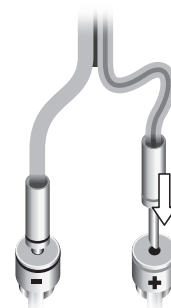
Optionaler Lautsprecherkabel-Anschluss mit Bananensteckern
