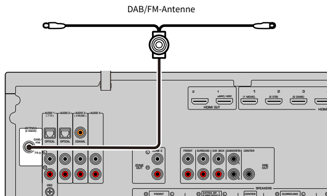
Gerät (Rückseite)
