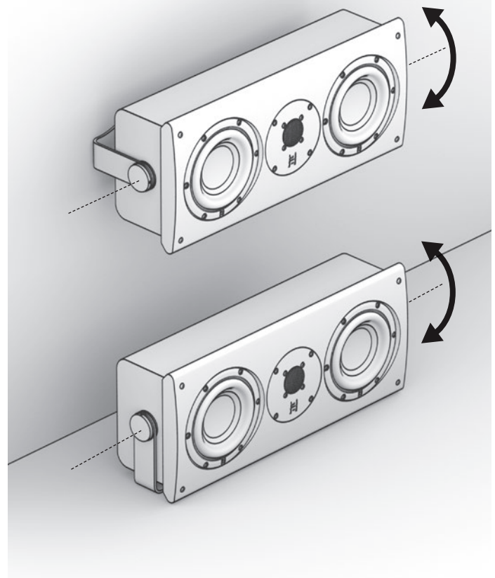
Schwenkpositionen waagrecht
