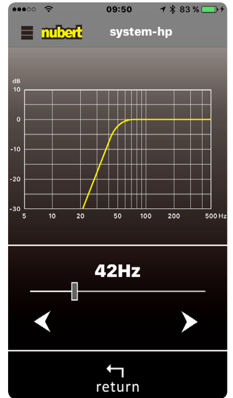
Mit dem Hochpassfilter kann die Basswiedergabe der X-3000 perfekt auf die Raumakustik angepasst werden
