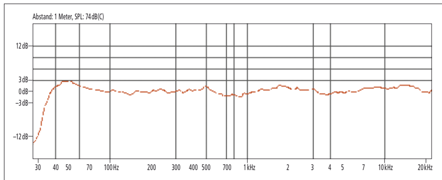
Unser Hörraum meint es im Bass sehr gut mit dem DSP-gestützten Aktivlautsprecher
