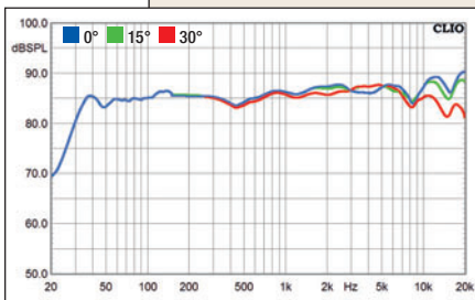
Frequenzgang Sensationeller Tiefgang bis unter 40 Hz und sehr linearer Frequenzverlauf
