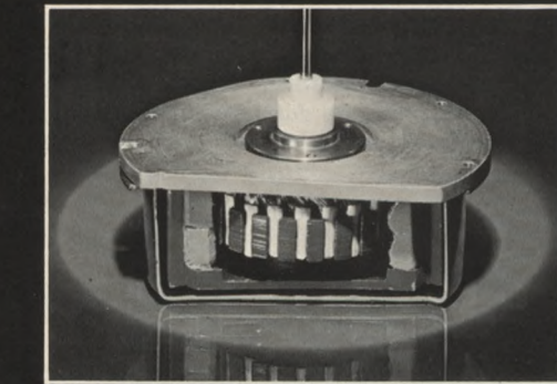
Direktantrieb-System mit 2 Motoren.
