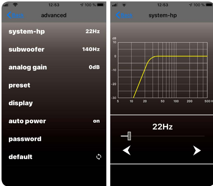
Dank umfangreicher Klangeinstellungen inklusive eines System-Hochpassfilters (rechts) wird der Klang perfekt auf Hörgeschmack und Raumakustik abgestimmt
