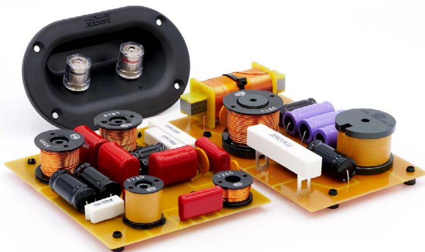
Die Frequenzweichen sämtlicher nuBoxx-Lautsprecher werden mit hochwertigen Passivbauteilen für eine optimale Klangqualität bestückt (Foto: Nubert)
